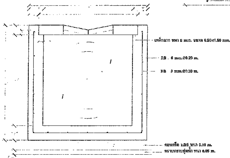
รูปตัดบ่อพัก A
