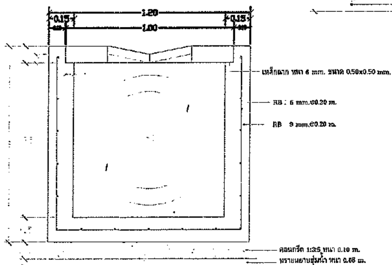
รูปตัดบ่อพัก A
