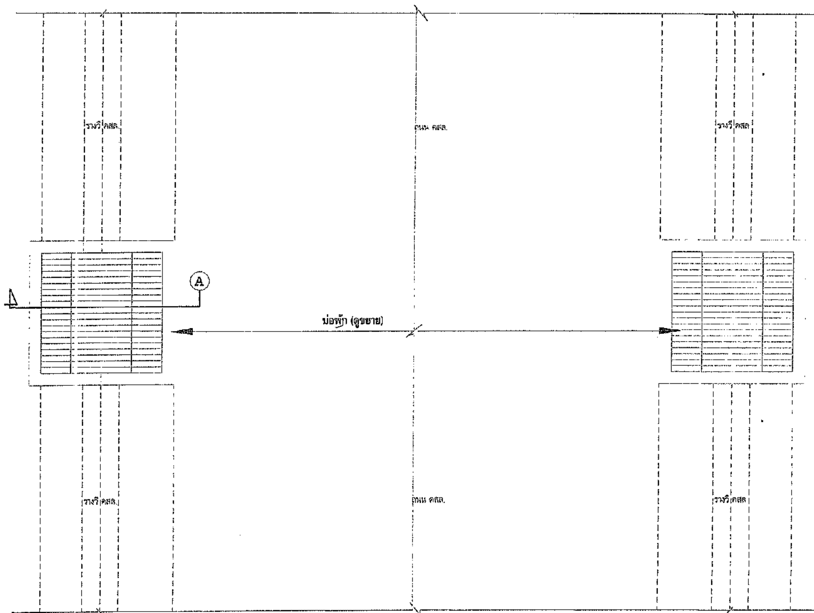
แปลนถนนรางวัด
