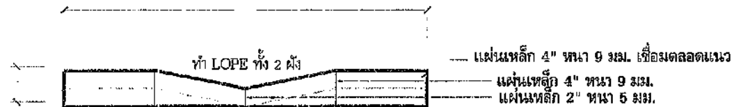
รูปตัดฝाप็อพักตะแกรงเหล็ก C
