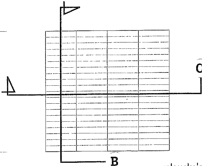
แปลนฝาบ่อพักตะแกรงเหล็ก
